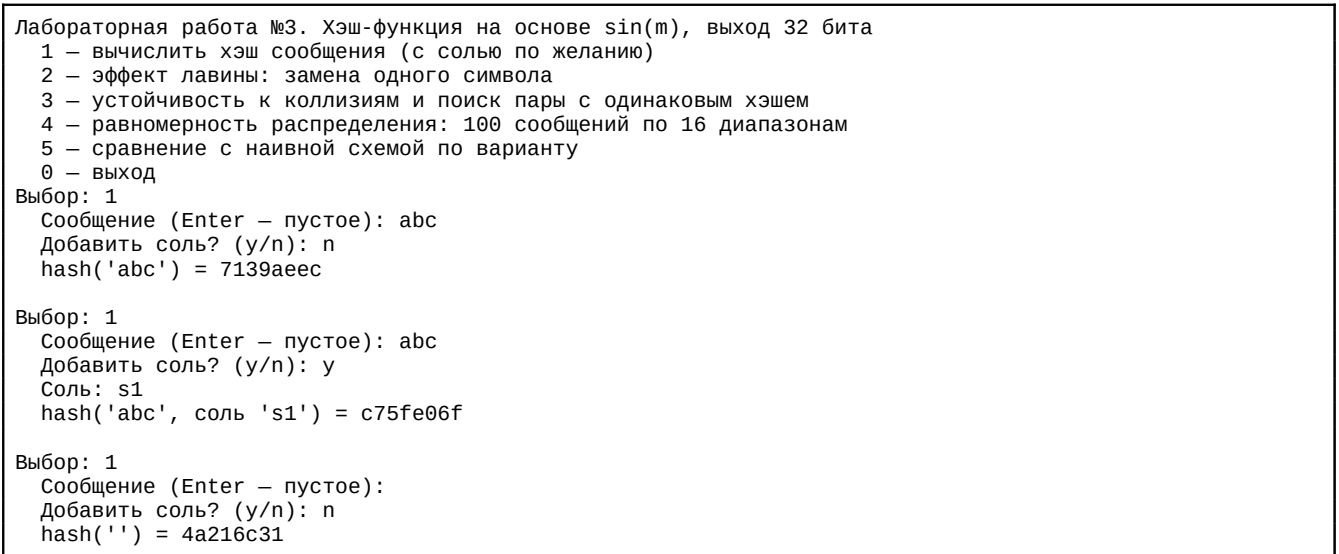
Рисунок 3.1 – Режим 1: хэш сообщения, хэш с солью, хэш пустого сообщения
