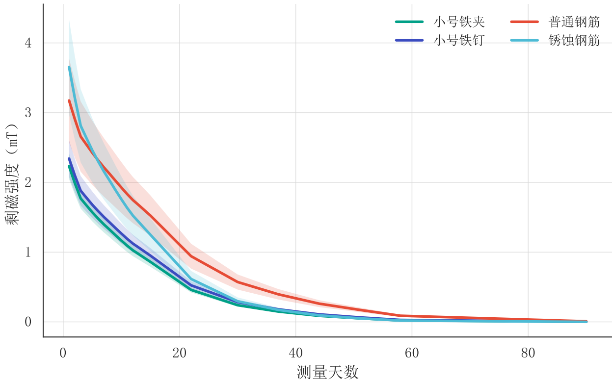
原始剩磁衰减曲线
