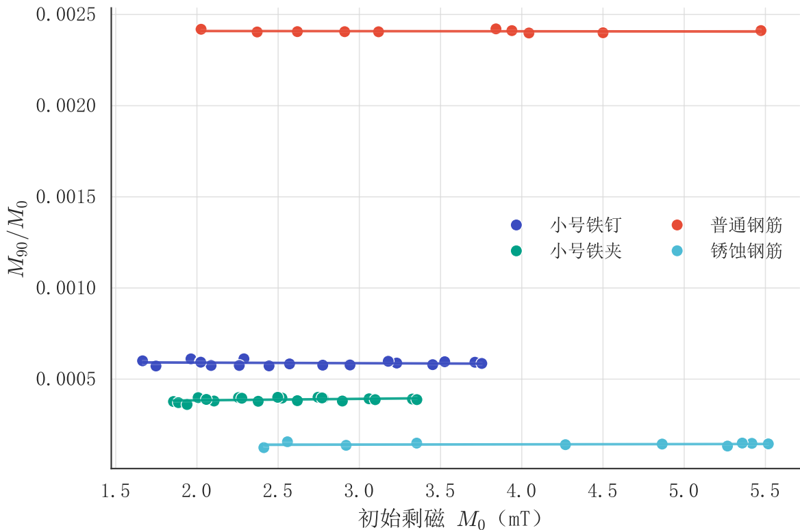
初始剩磁与 90 天保留率关系
