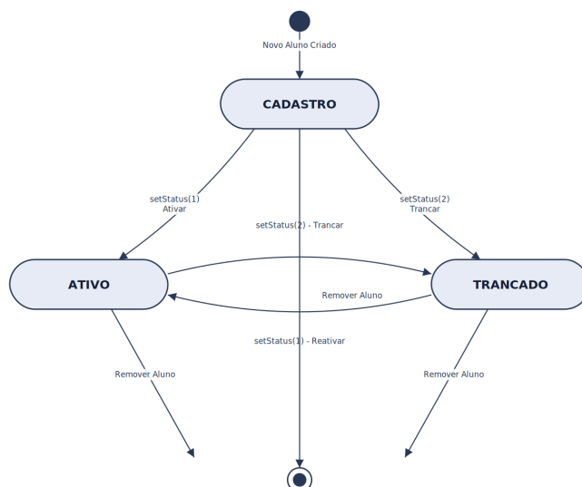
Figura 2 – Diagrama de máquina de estados do status de matrícula do aluno
