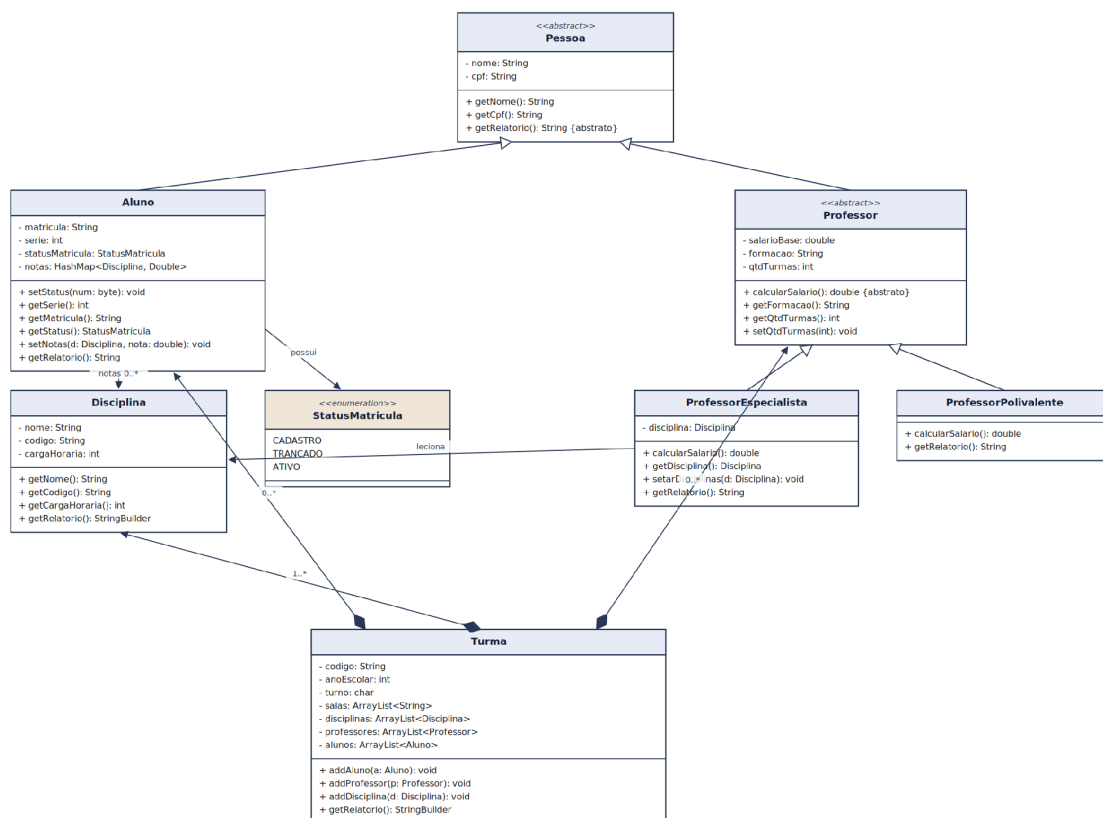
Figura 1 – Diagrama de classes do Sistema de Controle Escolar
