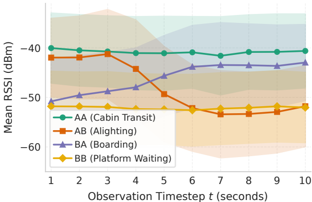
Mean RSSI Trajectory per Class ( \pm 1 \sigma )
