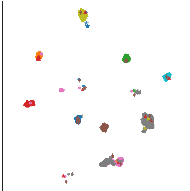
UMAP – CE+Triplet
