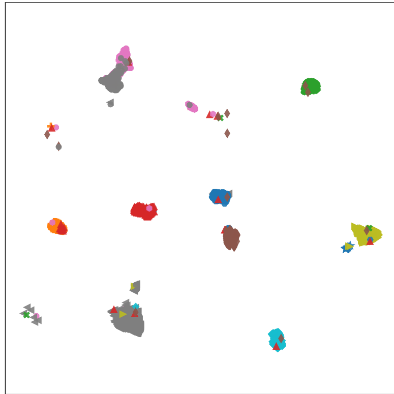
UMAP – CE
