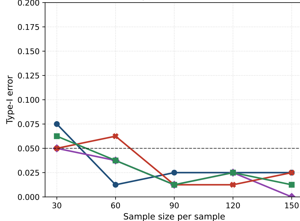
Type-I: B vs B
