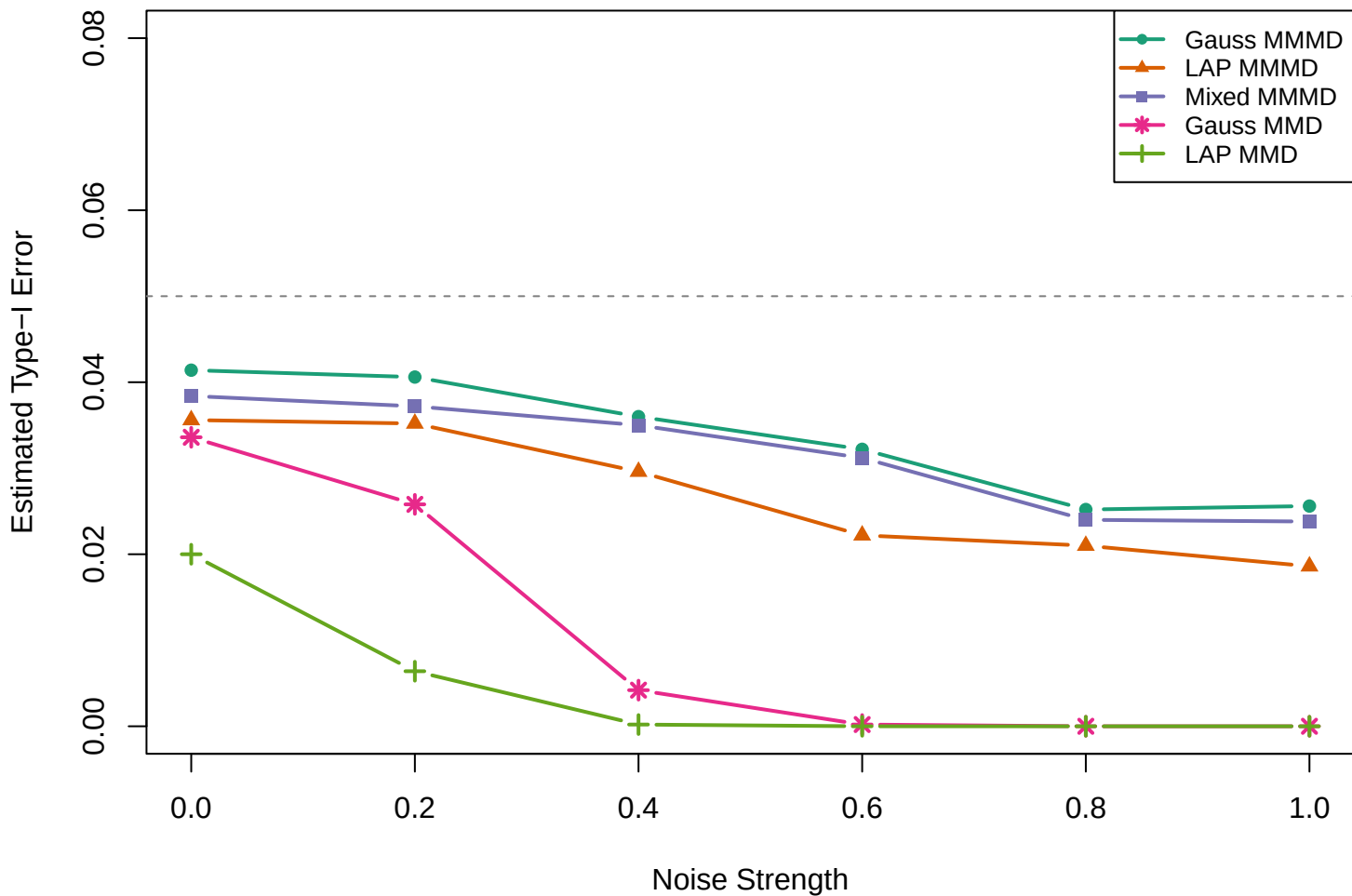
Type-I Error: {1,2,3} vs {1,2,3}
