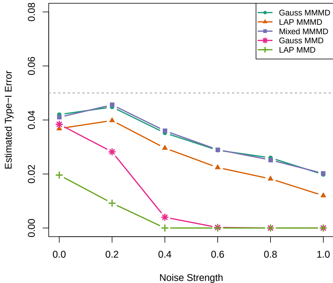
Type-I Error: \{1,2,8\} vs \{1,2,8\}
