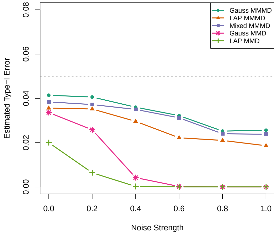
Type-I Error: \{1,2,3\} vs \{1,2,3\}
