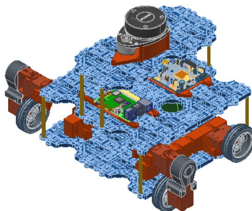
Rys. 2.5: Rzut izometryczny robota mobilnego z napędem Ackermana.
