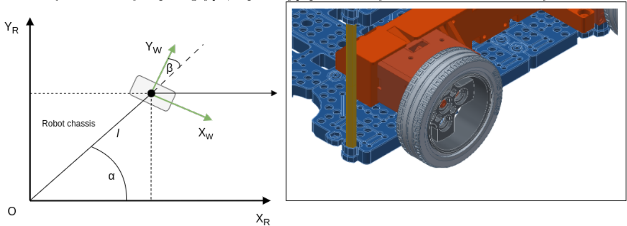
Rys. 1.2: Graficzne przedstawienie koła stałego w układzie robota.
