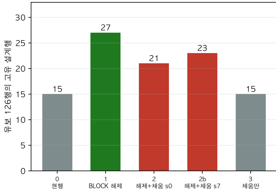
(a) 27 은 수집이 아니라 한 줄에서 나온다 — 채우면 오히려 내려간다
