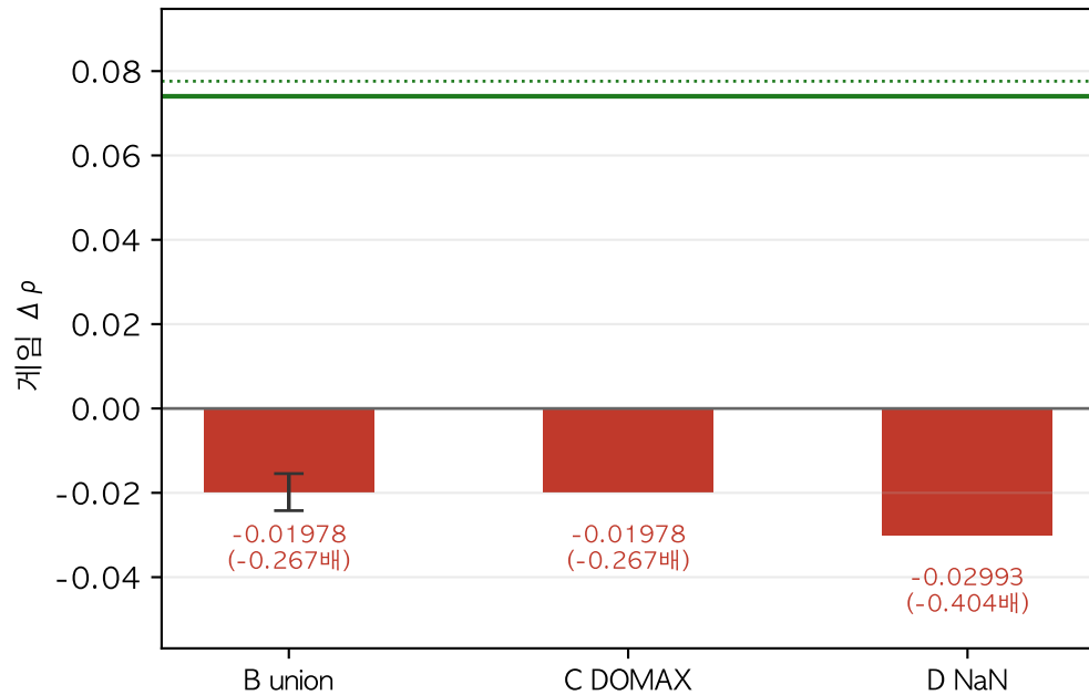
(b) 크기가 모자란 게 아니라 부호부터 반대다
