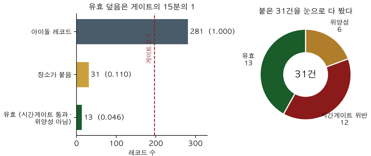
Figure 1: 덮음 31/281 = 0.110 (시군구이름 19 · 동이름 8 · city만 4). 그 31건을 눈으로 가르면 유효 13 · 시간 게이트 위반 12 · 위양성 6 이다.
