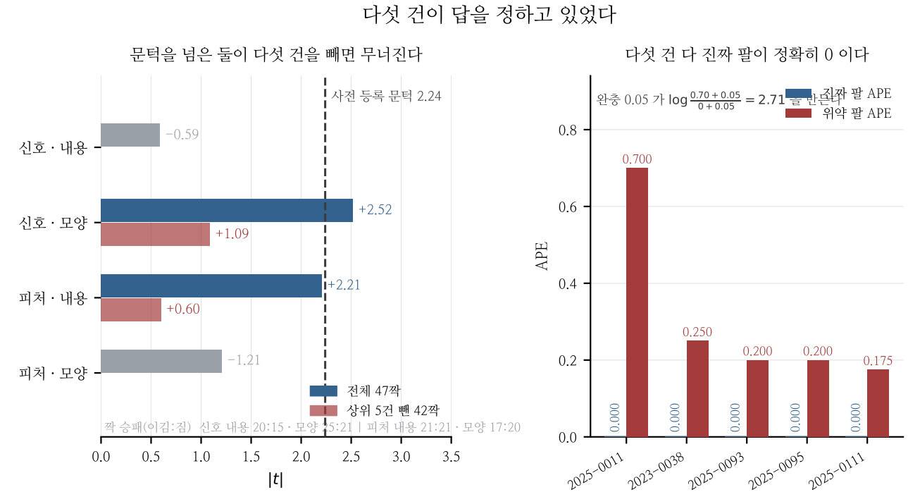
Figure 1: 왼쪽 — 네 비교의 |t| 와, 절대값 상위 다섯 건을 뺐을 때, 오른쪽 — 그 다섯 건.
