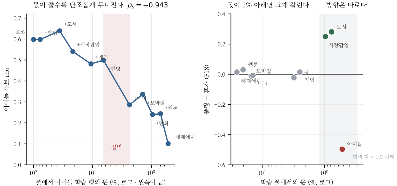
Figure 1: 왼쪽 — 폴을 작은 도메인부터 키우며 켜 아이들 유보 \rho . 오른쪽 — 다른 도메인들의 몫과 폴링 이득.
