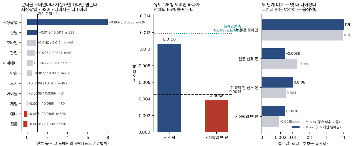
Figure 1: 왼쪽: 문턱을 도메인마다 계산하면 하나만 넘는다. 가운데: 유보 126행 도메인 하나가 판 신호 몫의 66% 를 만든다. 오른쪽: 두 단계 비교 — 넷 다 나아졌는데 판은 여전히 안 움직인다.
