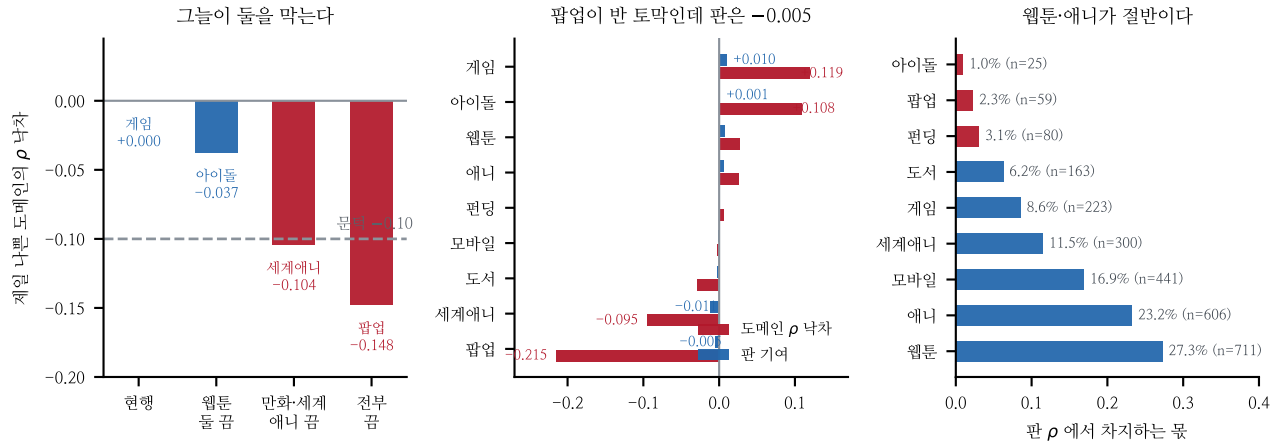
Figure 1: 왼쪽 — 그들이 둘을 막는다. 가운데 — 팝업이 반 토막인데 판은 -0.005 . 오른쪽 — 웹툰·애니가 절반이다.
