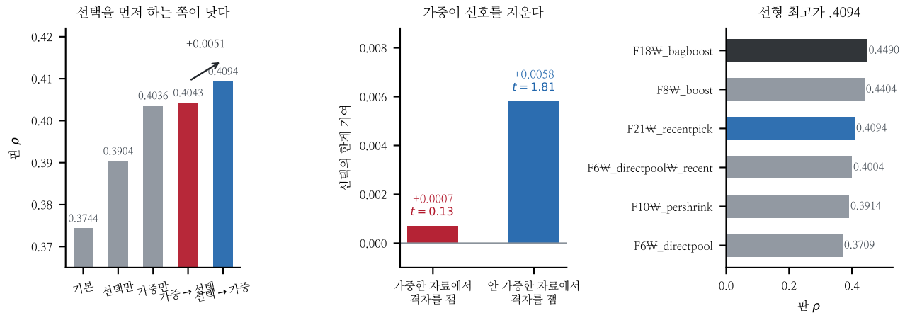
Figure 1: 왼쪽 — 선택을 먼저 하는 쪽이 낫다. 가운데 — 가중이 신호를 지운다. 오른쪽 — 선형 최고가 .4094.
