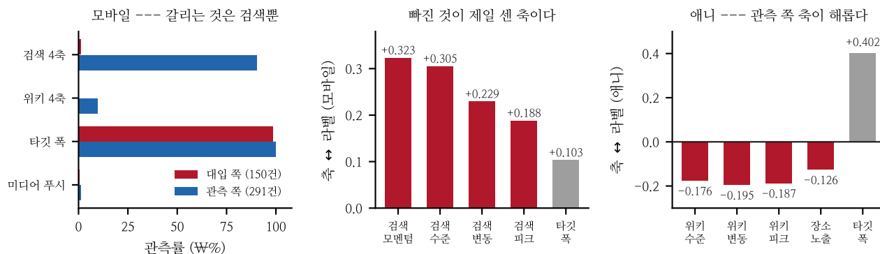
Figure 1: 왼쪽 — 모바일에서 갈리는 것은 검색뿐. 가운데 — 그 검색이 제일 센 축. 오른쪽 — 애니는 관측 쪽 축이 해롭다.
