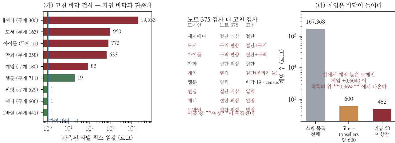
Figure 1: (가) 도메인별 관측 라벨 최소(원값, 로그축)와 자연 바닥 1. 초록 셋만 바닥에 닿는다. (나) 노트 375 판정과 고친 판정 — 아홉 중 여섯이 뒤집힌다. (다) 게임의 바닥 둘. 스텝 검색이 보고하는 167,368건에서 topsellers 앞 600을 받고, 다시 리뷰 50 미만을 잘라 482행이 남는다.
