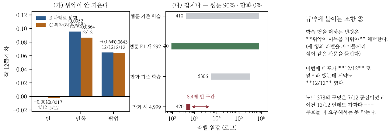
Figure 1: (가) 판 · 만화 · 팝업의 짝 12뽑기 차. 위약(주황)이 어디서나 실제 팔(파랑)을 따라온다. (나) 라벨 범위. 웹툰 E1은 기존 학습과 겹치고 만화의 새 행은 8.4배 떨어진 별개 구간이다. (다) 규약에 붙이는 조항.
