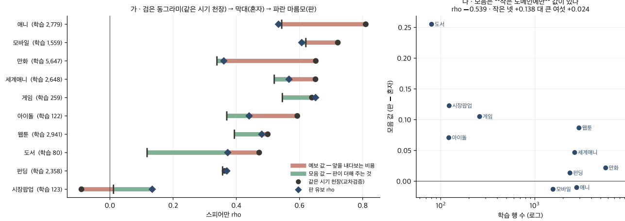
Figure 1: 가 — 도메인마다 검은 동그라미(같은 시기 천장)에서 붉은 막대만큼 떨어져 혼자 예보에 이르고, 초록 막대만큼 올라 판에 이른다. 붉은 막대가 거의 어디서나 길다. 나 — 모음 값은 학습 행 수와 반대로 간다( \rho = -0.539 ). 도서 80행에 +0.2551, 만화 5,647행에 +0.0217.
