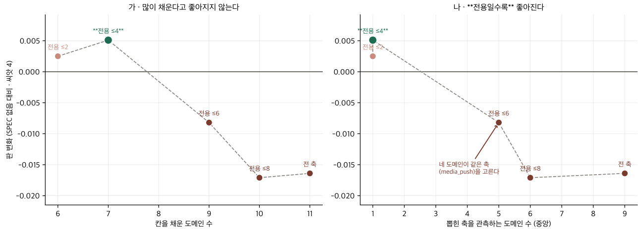
Figure 1: 같은 다섯 점을 두 축으로 놓았다. 가 — 채움과 판 사이엔 관계가 없다(붕우리를 지나 내려간다). 나 — 뽑힌 축이 얼마나 전용이냐와는 깨끗하게 단조다.
