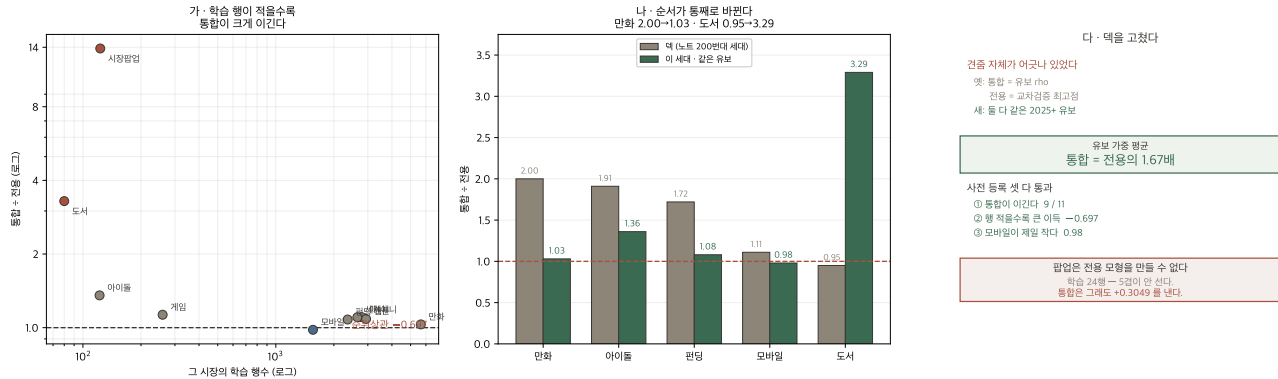
Figure 1: 가 — 학습 행이 적을수록 크게 이긴다. 나 — 순서가 뒤집힌다. 다 — 텍을 고쳤다.
