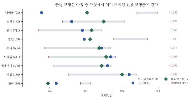
Figure 1: 도메인마다 섞음(과적합 바닥) → 속천장 구간, 그 안에 지금(파랑)과 유보 안 CV(초록). 초록이 파랑 왼쪽이면 여지가 음수다.
