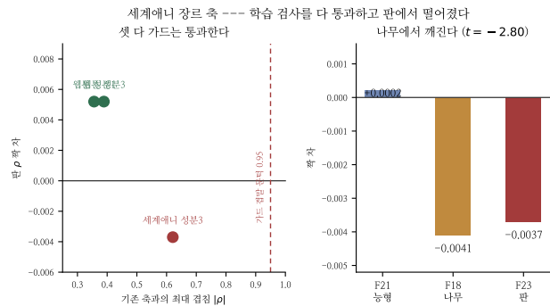
Figure 1: 원쪽 — 겹침과 판 이득. 셋 다 가드 문턱 왼쪽이다. 오른쪽 — 세계애니 축이 어디서 깨지나.
