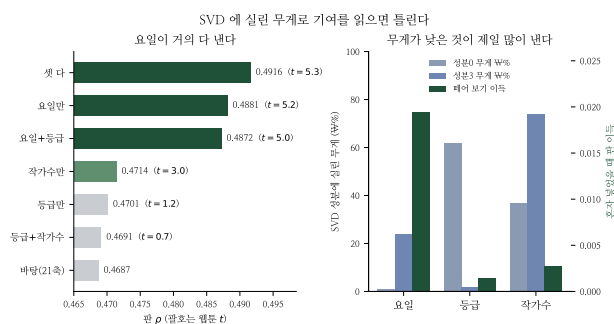
Figure 1: 왼쪽 — 토큰 무리를 떼어 넣어 본 판. 오른쪽 — SVD 무게와 실제 기여가 어긋난다.
