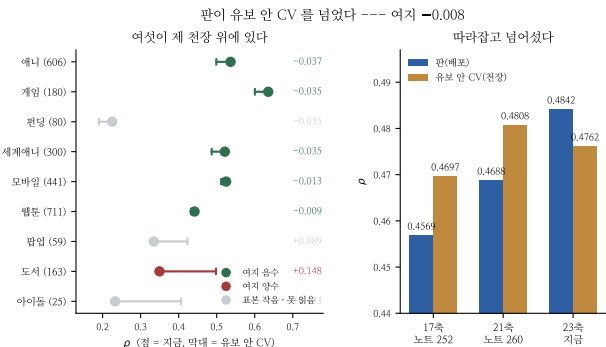
Figure 1: 왼쪽 — 도메인마다 지금(점)과 유보 안 CV(막대). 오른쪽 — 세 걸음.
