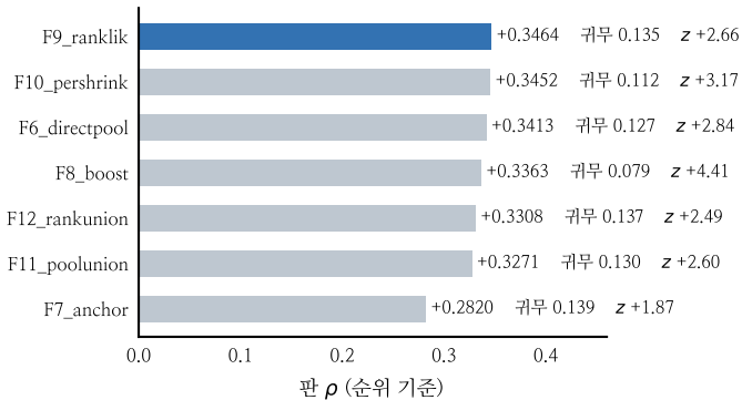
순위는 \rho , z 는 가드
