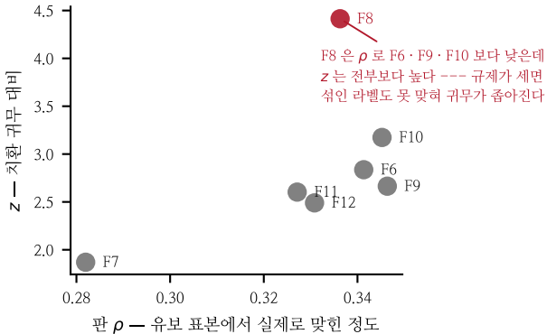
z 순위와 \rho 순위가 어긋난다
