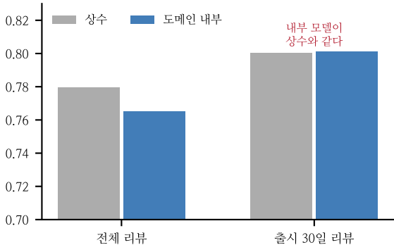
평균절대오차
