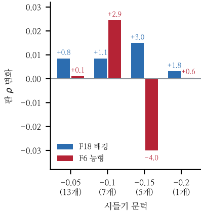
한 칸 옆에서 부호가 뒤집힌다
