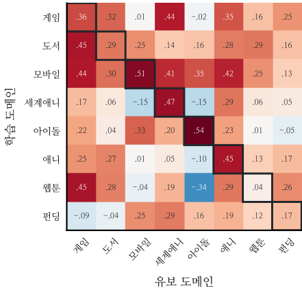
대각선이 늘 이기지 않는다
