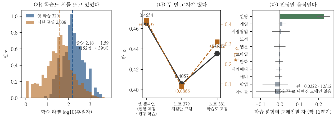
Figure 1: (가) 옛 학습 320건과 더한 균일 2,038건의 라벨 분포. 중앙이 2.182 → 1.591(log10), 곧 후원자 152명 → 39명이다. (나) 두 노트의 궤적 — 채점만 고치면 판이 떨어지고 학습까지 고치면 대부분 돌아온다. (다) 학습 넓힘의 도메인별 차(딱 12뽑기, 막대는 딱 SD). 편딩만 크게 움직이고 나머지 열은 0 근처다.
