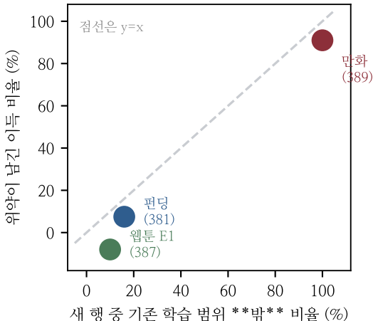
(나) 밖이 곧 잔량이다 (n=3)
