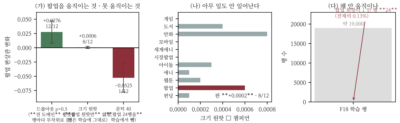
Figure 1: (가) 팝업을 움직이는 조작과 못 움직이는 조작. 제 원하트만 없애는 것은 아무것도 안 한다. (나) 열한 도메인 전부 |r| \leq 0.0008 . (다) 팝업 원하트 1인 학습 행은 24 — 전체의 0.13%.
