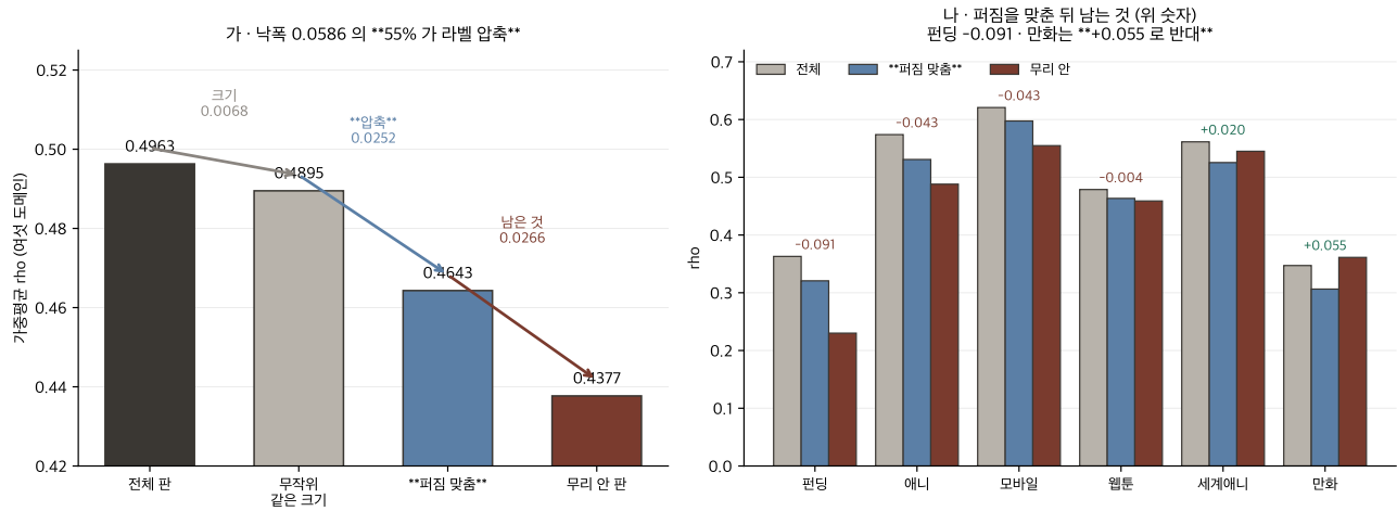
Figure 1: 가 — 낙폭의 세 조각. 나 — 퍼짐을 맞춤 뒤 도메인마다 남은 것.
