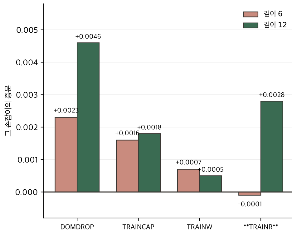
나 · **깊이 감응은 손잡이마다 다르다** DOMDROP 2 배 · TRAINR 0 → 전부
