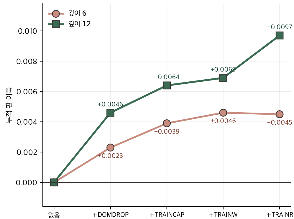
가 · 누적 --- 깊이 12 가 **0.0097** , 깊이 6 은 0.0045
