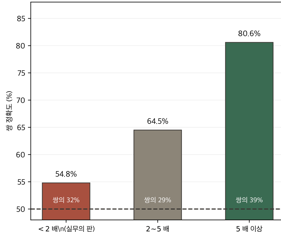
나 · 네 채택을 다 합쳐도\ < 2 배는 54.8 → 55.0
