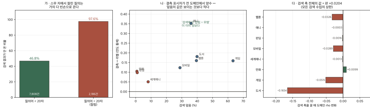
Figure 1: 가 — 스무 자 절벽. 나 — 결측이 정보다. 다 — 덮음과 값이 안 맞는다.
