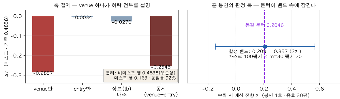
Figure 1: 왼쪽: 축 절제 — venue 단독 \Delta -0.286 이 동시 마스크 -0.254 를 단독으로 다 설명한다. 오른쪽: 합성 밴드와 문턱.
