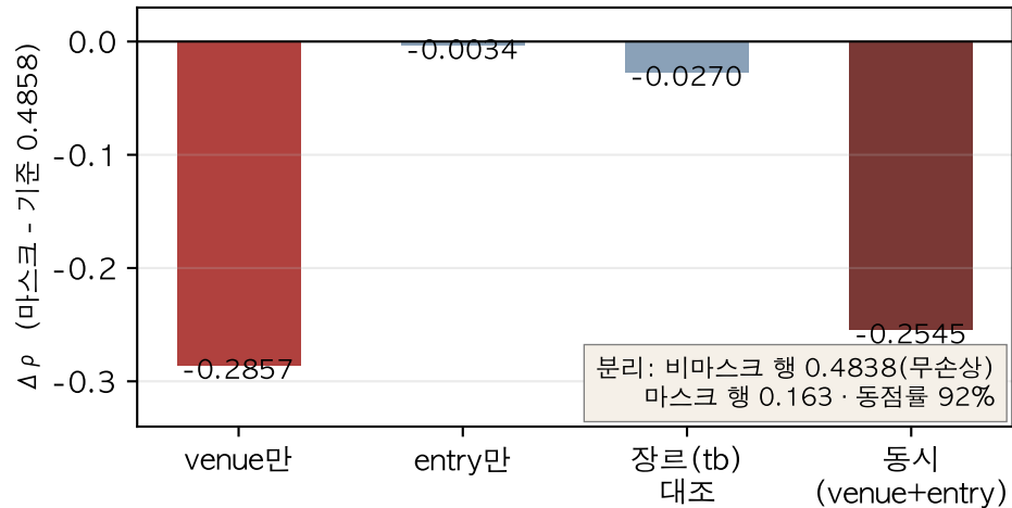
축 절제 — venue 하나가 하락 전부를 설명
