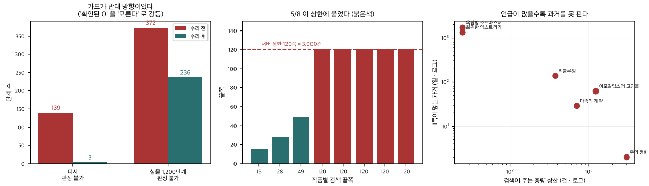
Figure 1: 왼쪽: 가드를 바로 걸자 판정 불가가 무너진다. 가운데: 여덟 작품 중 다섯이 서버 상한(120쪽 = 3,000건)에 붙었다. 오른쪽: 검색이 주는 총량이 많을수록 1쪽이 덮는 과거가 짧다 — 말이 많을수록 못 판다.
