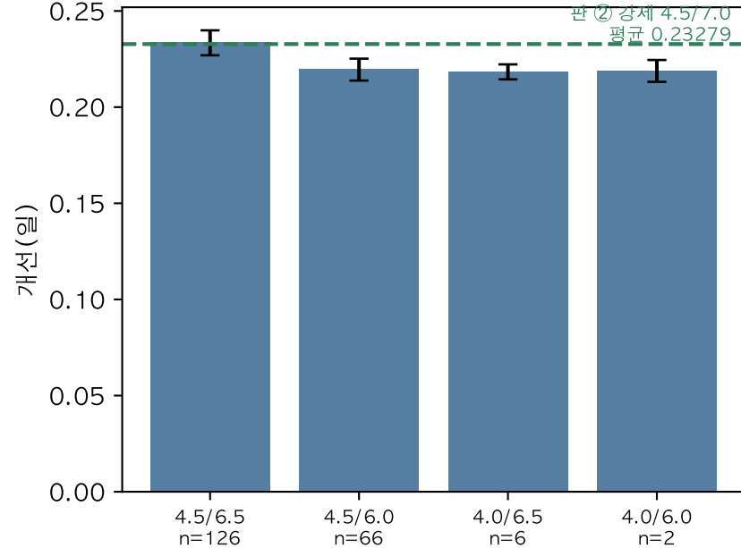
(c) 귀무의 prevmed 경계 상태 진짜는 (4.5, 7.0) — 200뽑기가 한 번도 안 가는 자리
