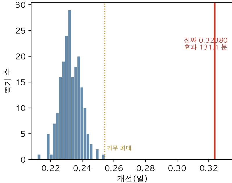
(b) 판 ② 달력제거 + 경계 강제 경계 상태 1개 · k=0/200 · p=0.004975
