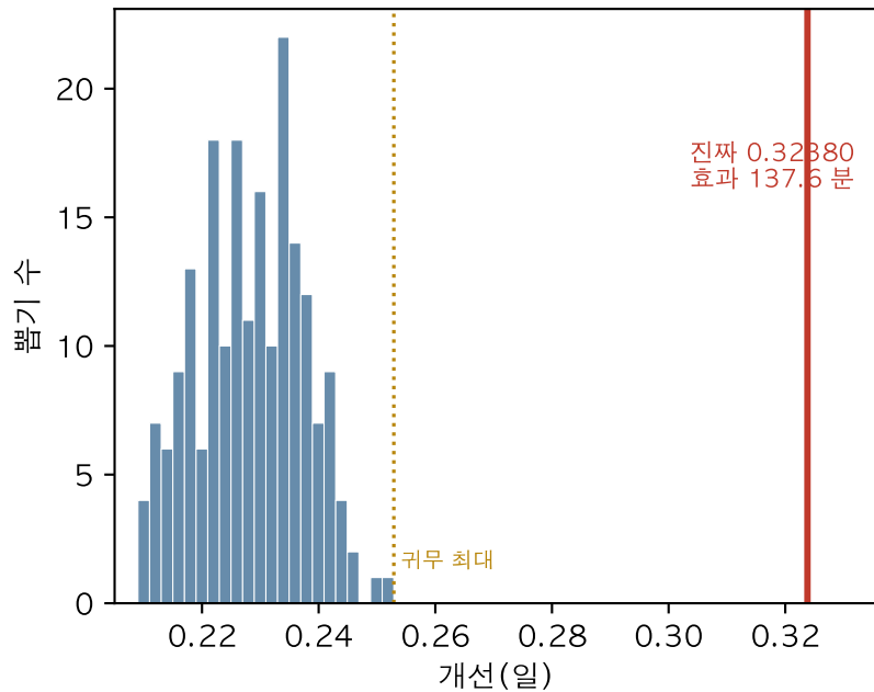
(a) 판 ① 달력제거 경계 상태 4개 · k=0/200 · p=0.004975
