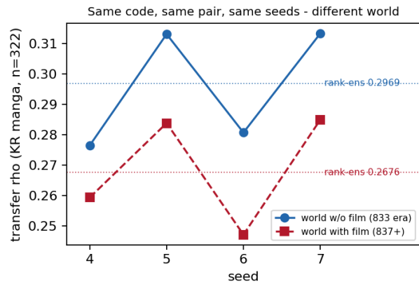
Figure 1: 같은 코드·같은 짝·같은 씨앗, 다른 세계. 영화 합류 전 (파랑) 씨앗별 전이 \rho 는 4/4 모두 합류 후(빨강)보다 높고, 순위평균 앙상블은 0.2969 → 0.2676으로 움직인다. 병기 관측: 영화 합류가 KR 만화 A-경로 전이를 \sim 0.03 낮췄다(SE 없음 — 주장 아님).
