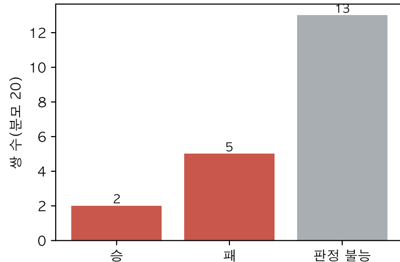
(c) 참 귀무끼리 짝지어도 7/20 = 35\% 가 「유의」 → 판정의 근거는 짝지은 구간이 아니라 순열 p 다
