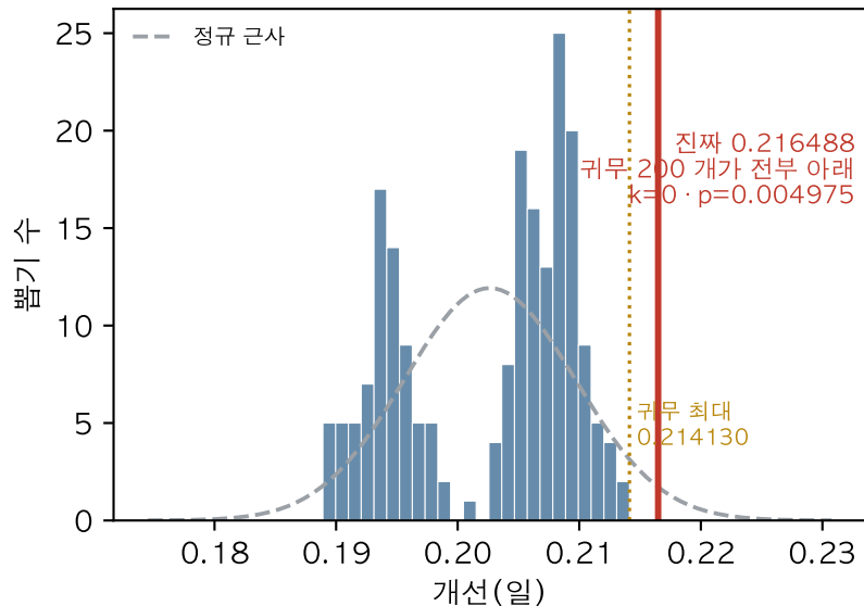
(a) 순열 200뽑기 — 꼬리가 정규보다 짧다 초과점도 -1.36 \cdot 표준화 최대 1.63 SD
