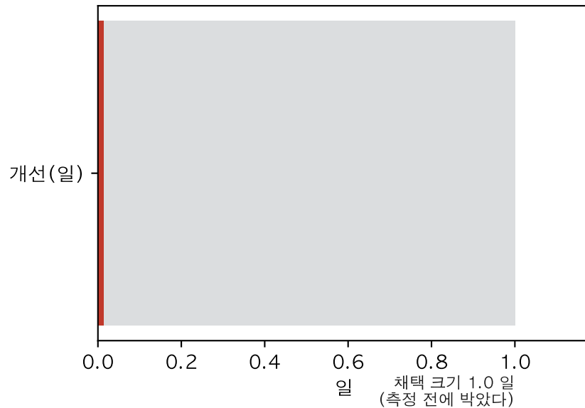
실측 0.0139 일 = 19.9 분 (b) 유의성과 크기는 둘이다 p=0.004975 로 이기고 72.2 배 모자라서 졌다
