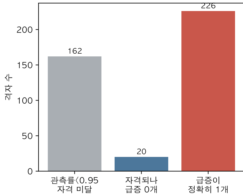
(a) 408 개 격자의 정체 홀드아웃 2,685 - 간격 있는 2,277 = 408 (15.20%)
