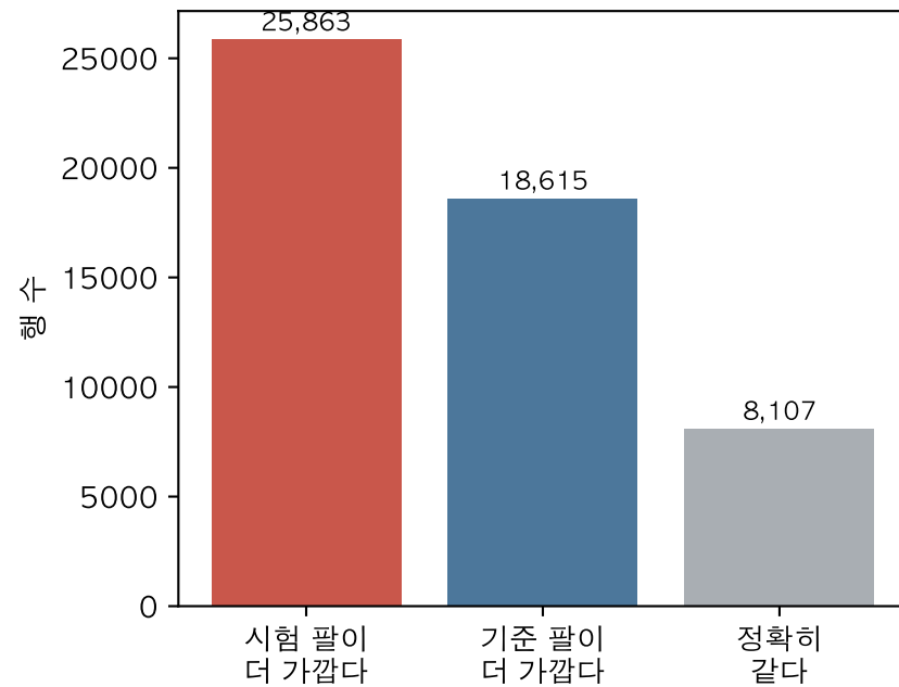
(b) 행으로는 순 7,248 행이 좋아졌다(분모 52,585) 그런데 MAE 10.3807 → 10.1642, 반올림하면 둘 다 10 일
