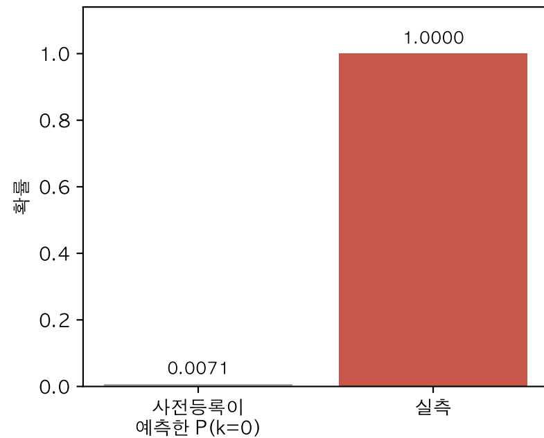
(c) 자기 적발 — 검출력 계산이 정규 근사 위에 서 있었다 정규 기대 k=4.88 · 실측 k=0 → 다음부터 경험분포로
