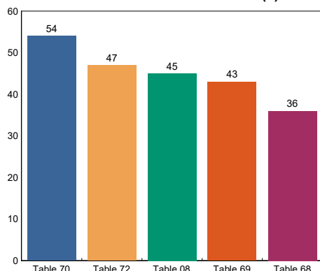
DEFECTOS 2DO TURNO TOP(5)
