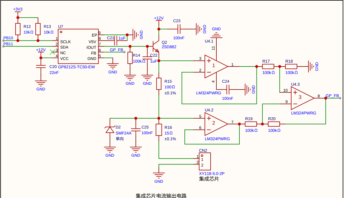
集成芯片电流输出电路
