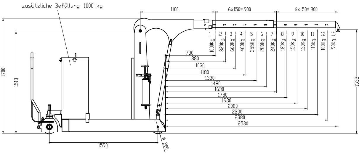
Eigengewicht des Krans: 365 kg
