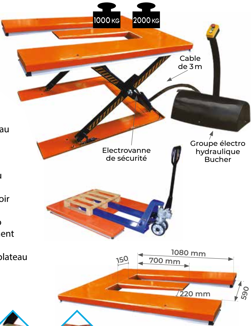
CADRE DE SÉCURITÉ ANTI-ÉCRASEMENT
