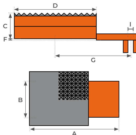
Exemple d'assemblage PC40 + RS40
