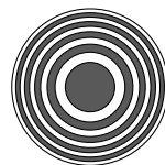
(a) 挡住奇数波带
